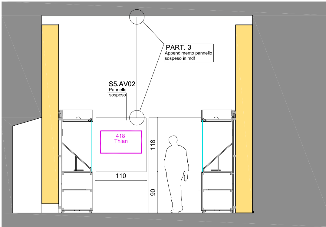
Parete 4
