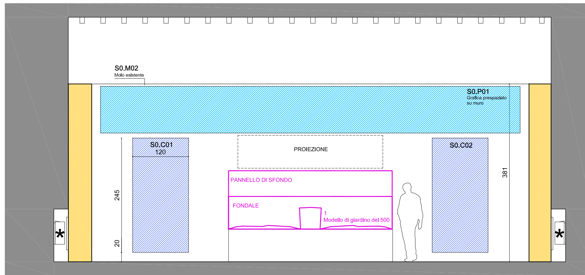
Parete 2
