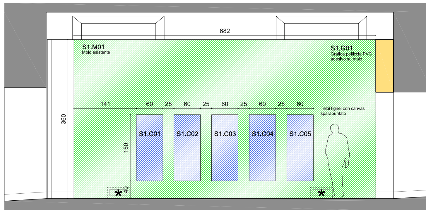
Parete 1
