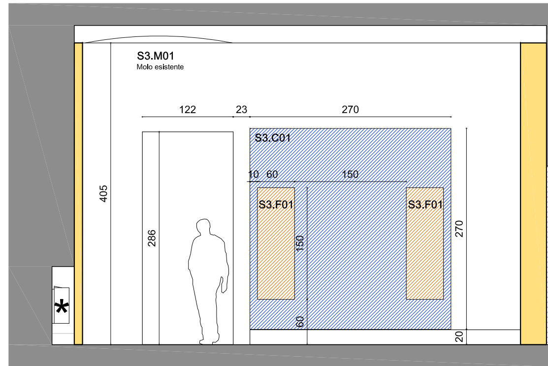
Parete 1
