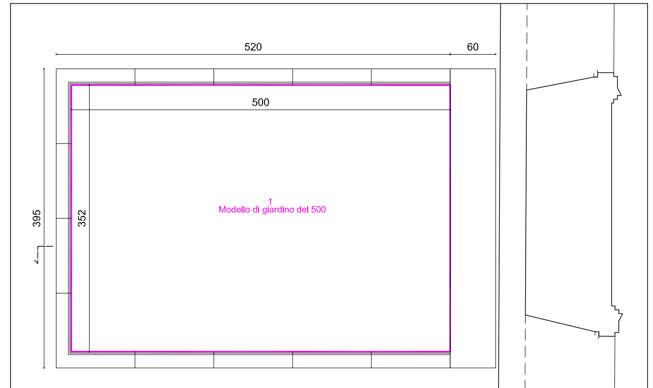
PIANTA
