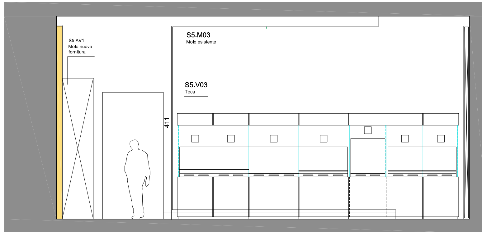
Parete 3
