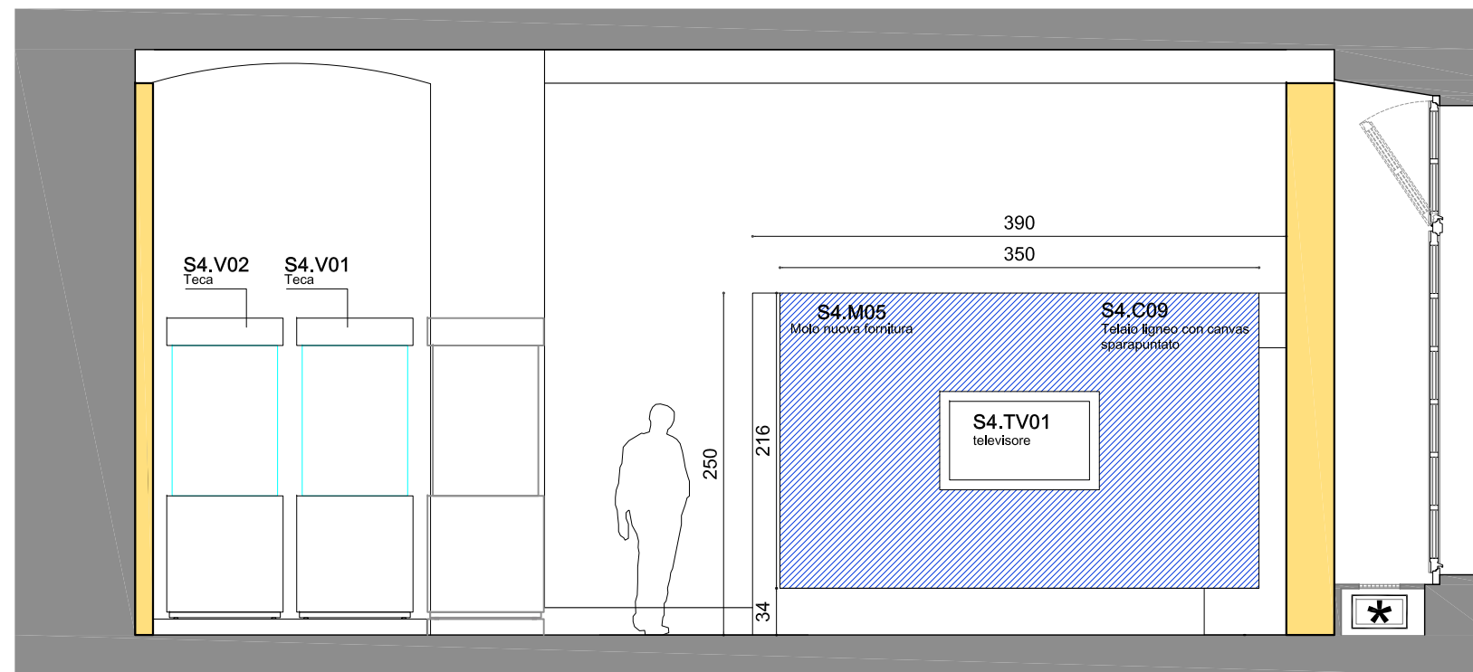
Parete 6
