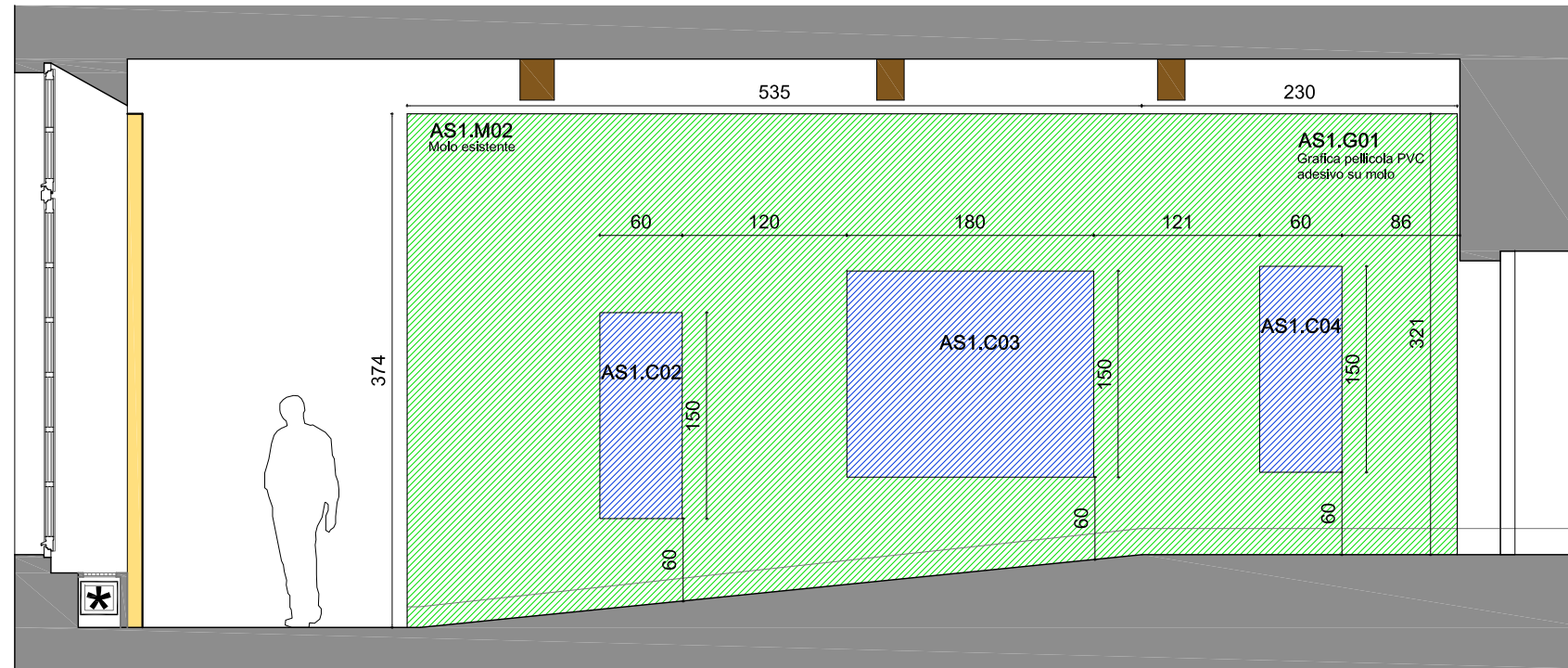
Parete 5
