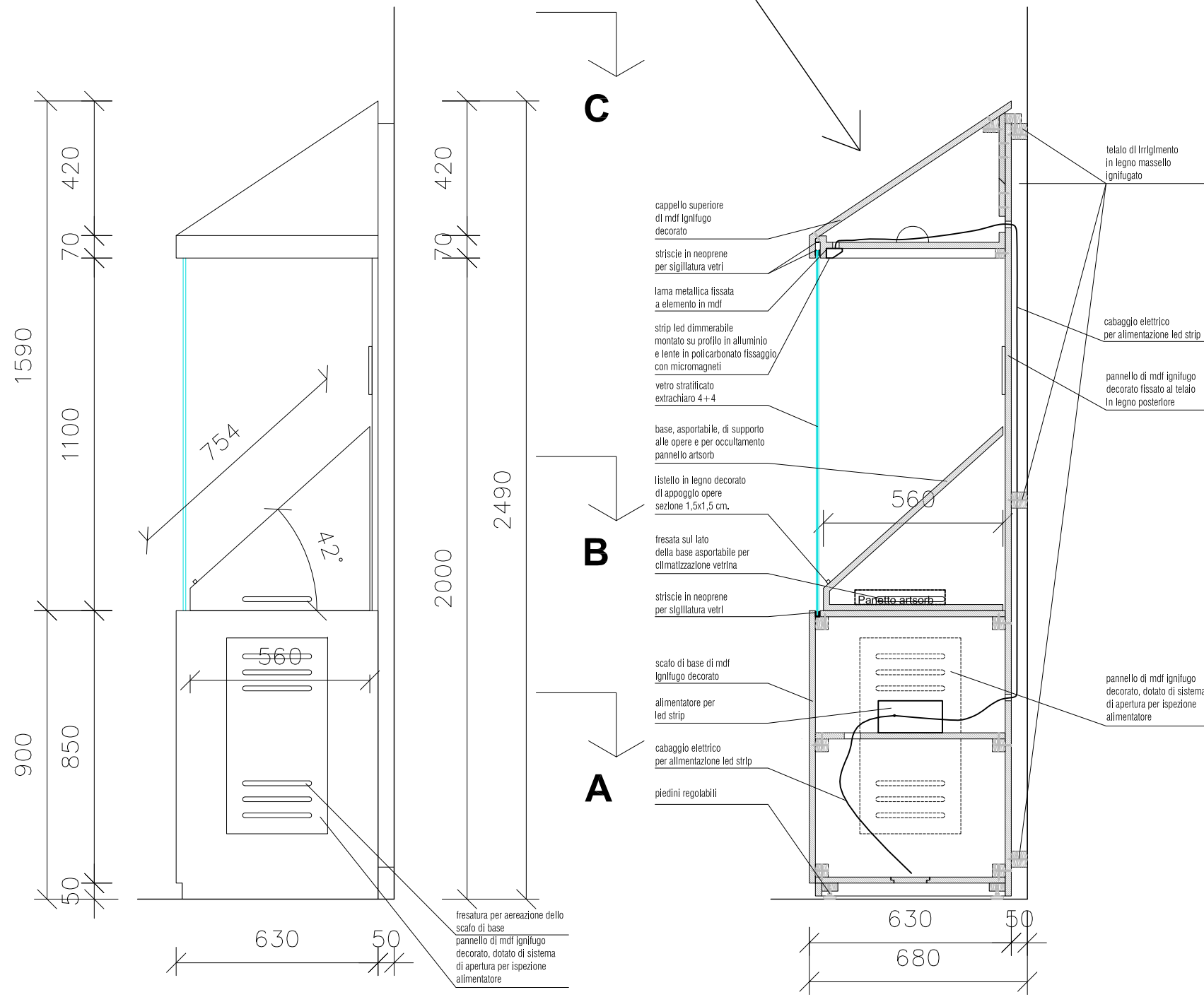
PROSPETTO LATERALE
