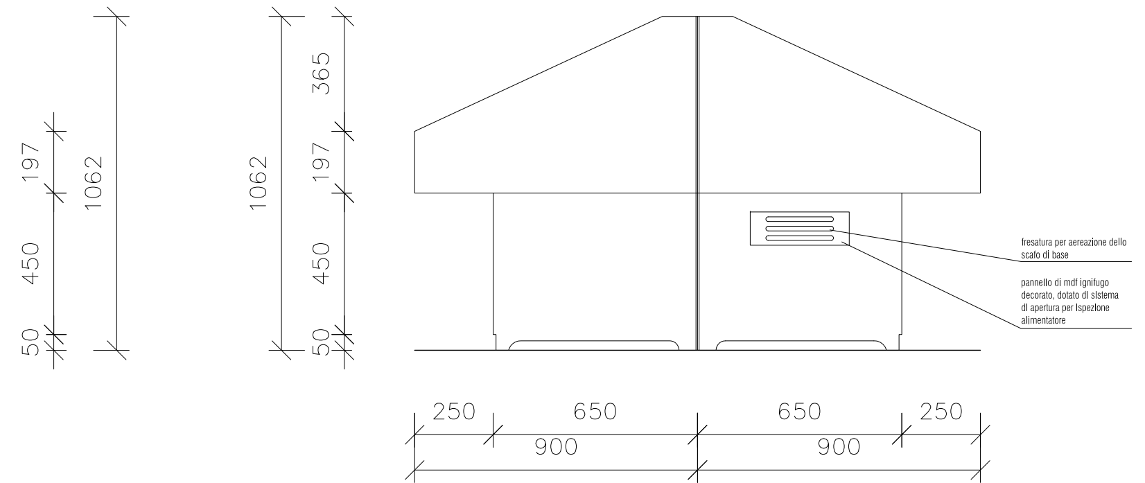
PROSPETTO LATERALE
