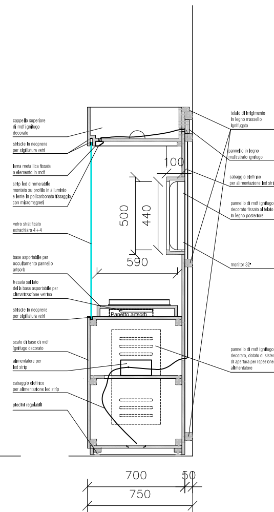
SEZIONE D
