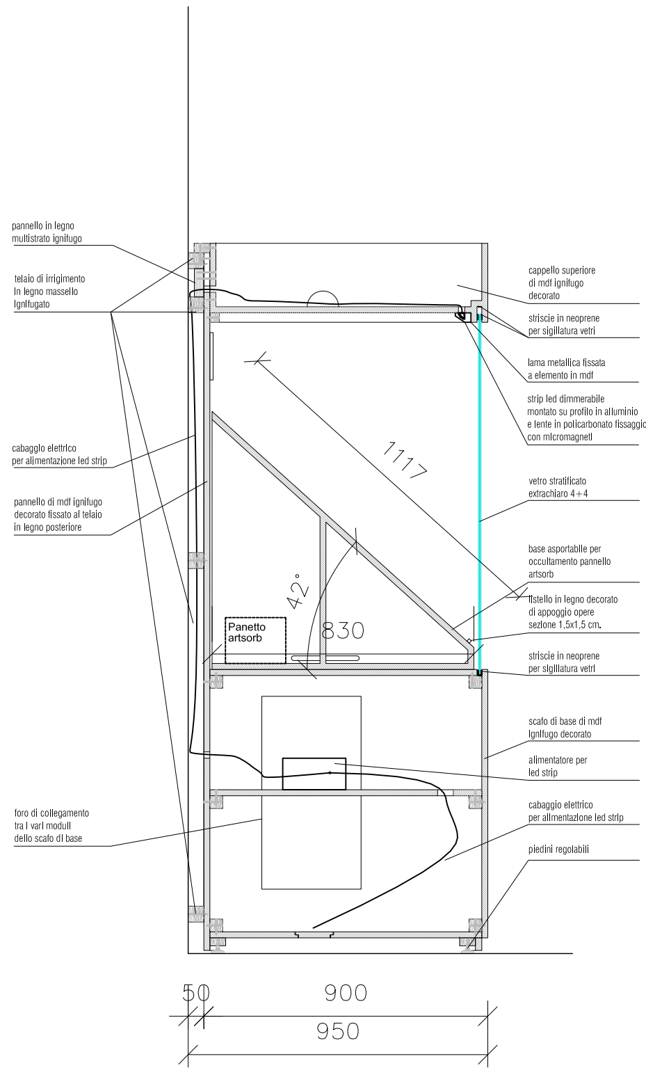
SEZIONE E
