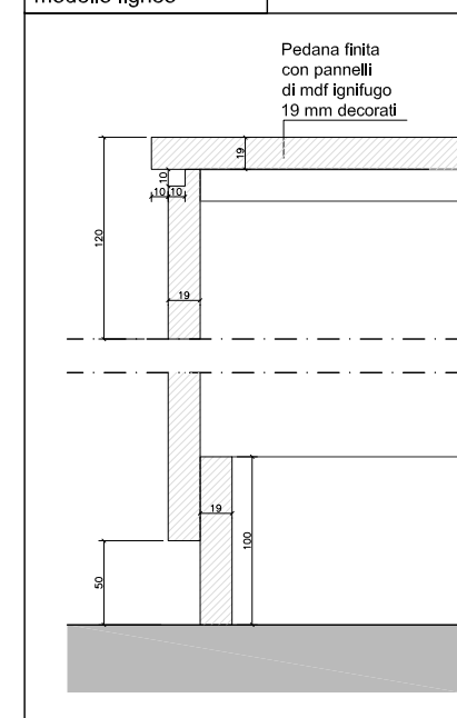
PART. 1 finitura supporti modello ligneo
