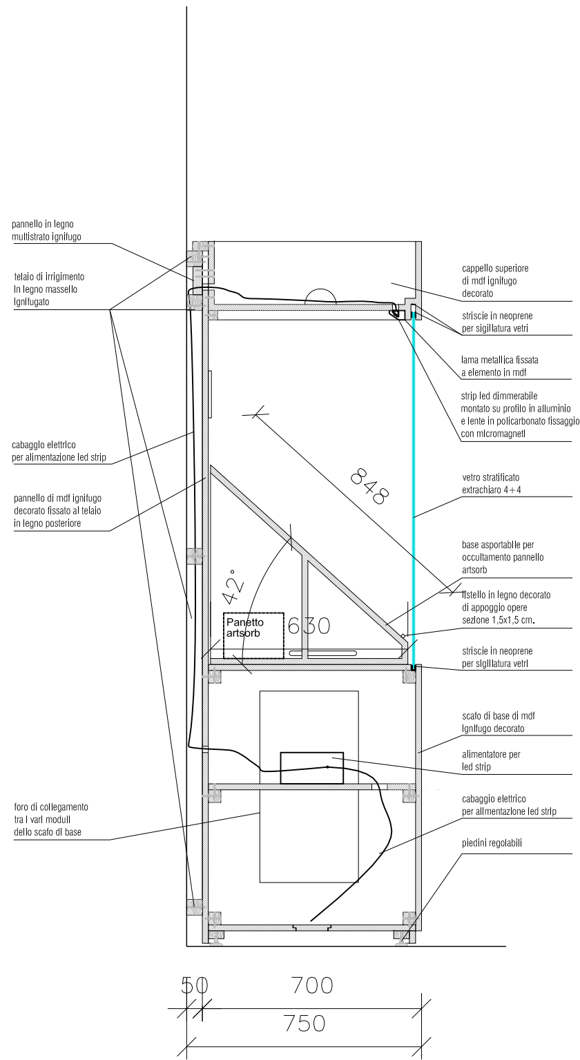
SEZIONE D
