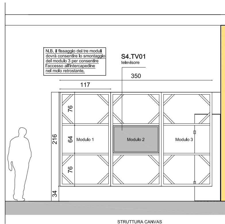
S4.C09 Telaio ligneo sparapuntato con telo grafico realizzato in masselli di legno ignifugato
