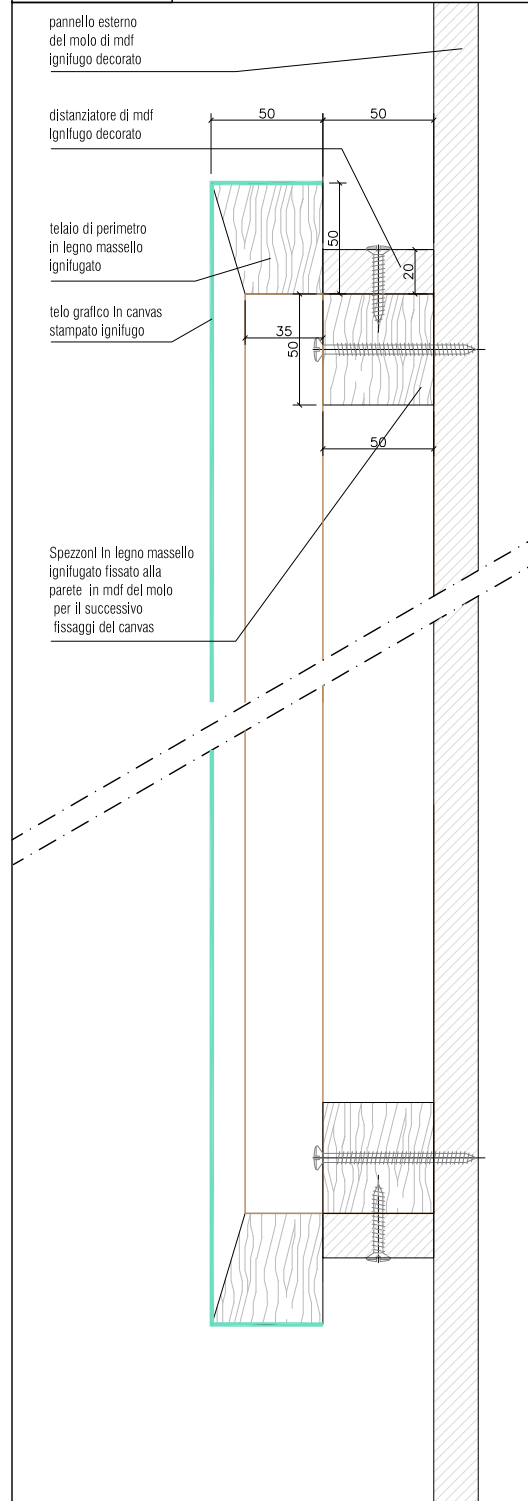
PART. 1 Fissaggio canvas alla parete in mdf del molo
