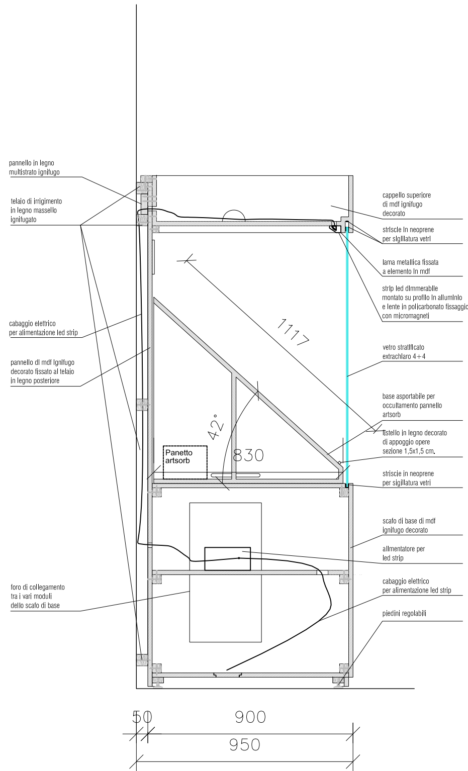
SEZIONE E
