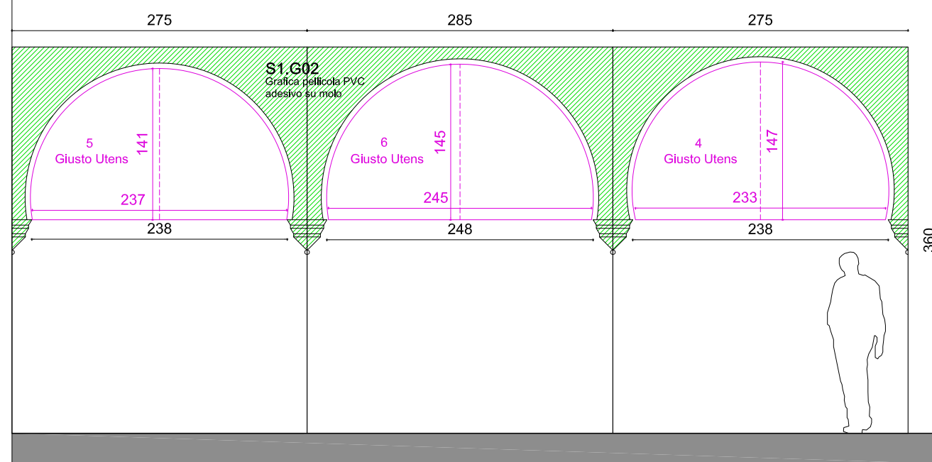
Sviluppo parete 3
