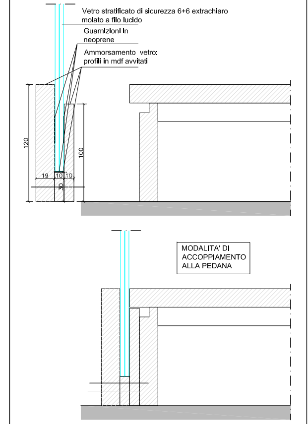
PART. 2 modalità di fissaggio vetri alla pedana
