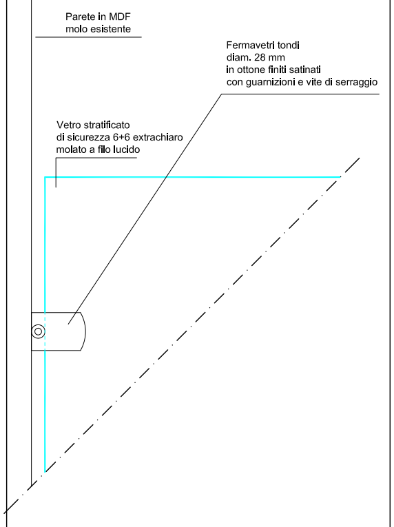
PART. 3 modalità di fissaggio vetri al muro
