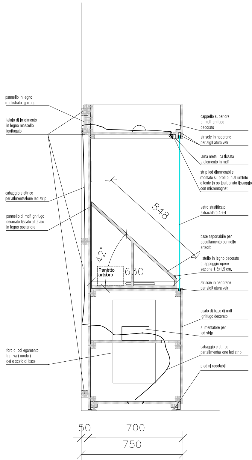
SEZIONE D
