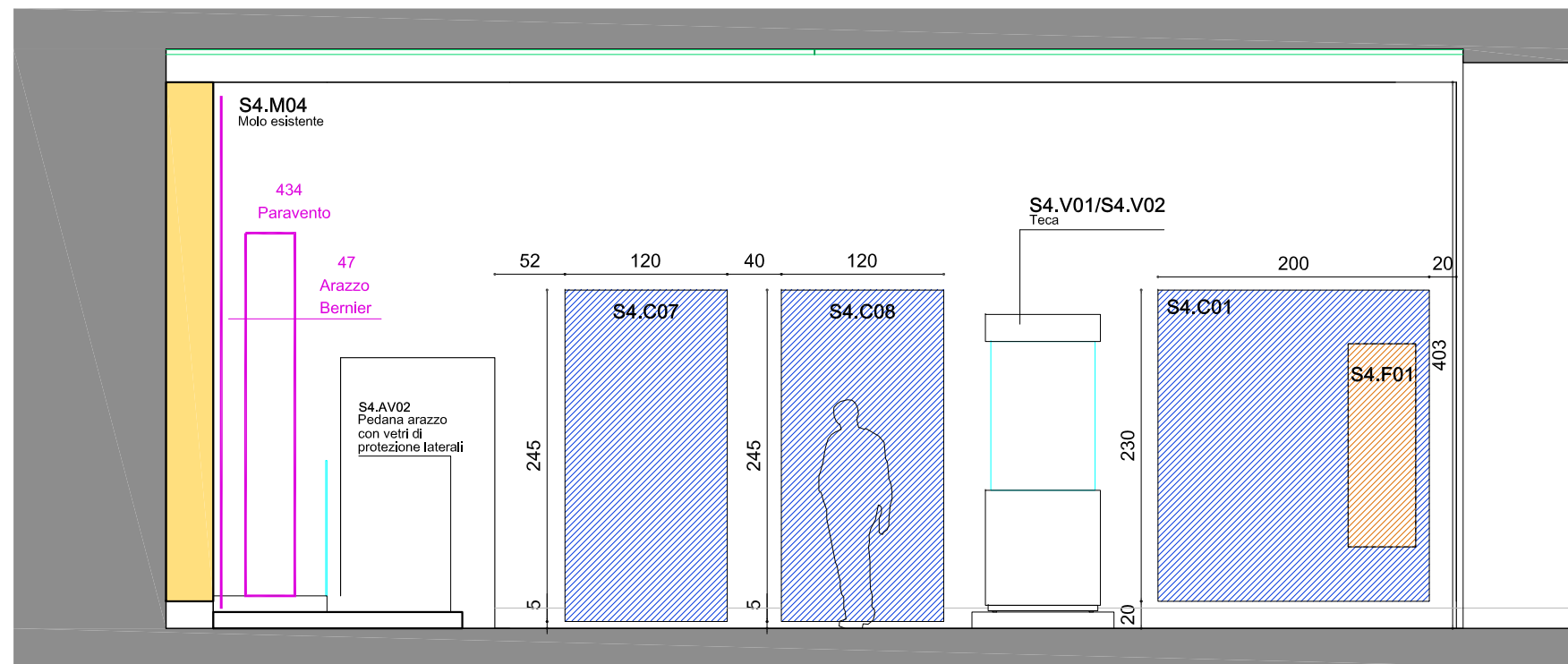
Parete 4
