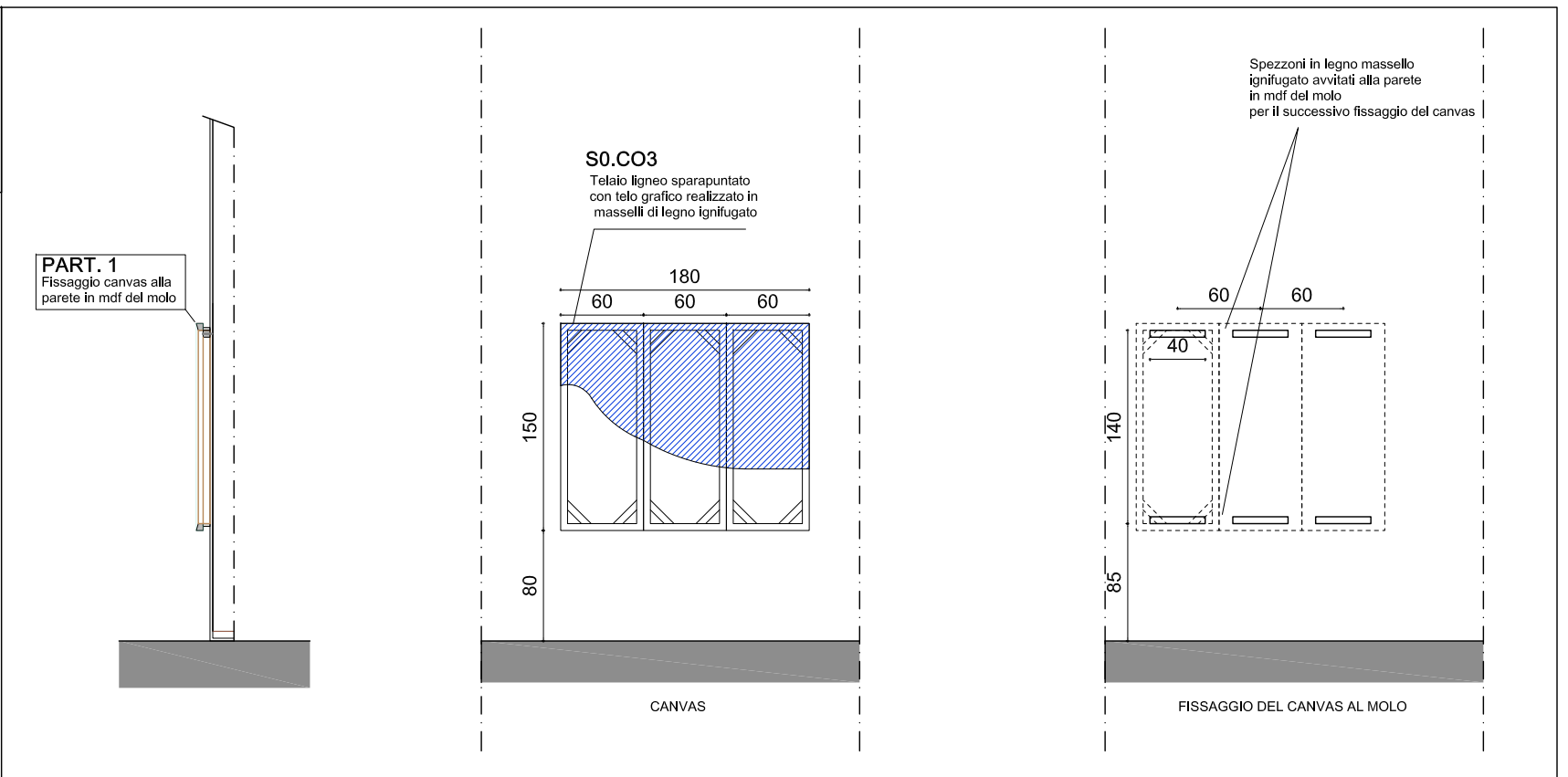
S0.CO3 Telaio ligneo sparapuntato con telo grafico realizzato in masselli di legno ignifugato
