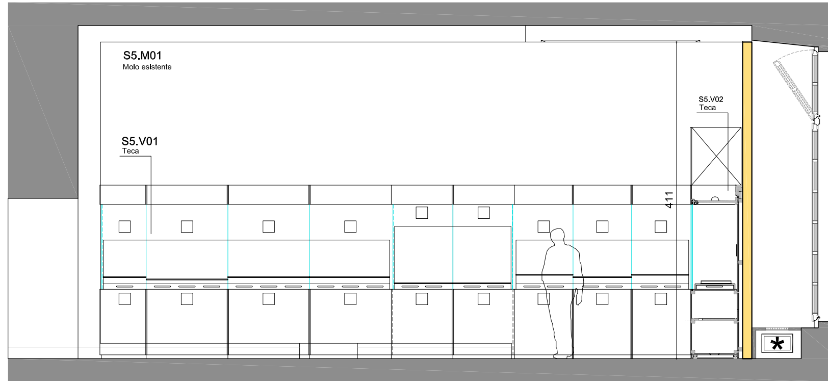
Parete 1
