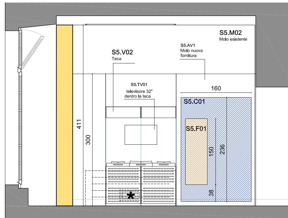
Parete 2
