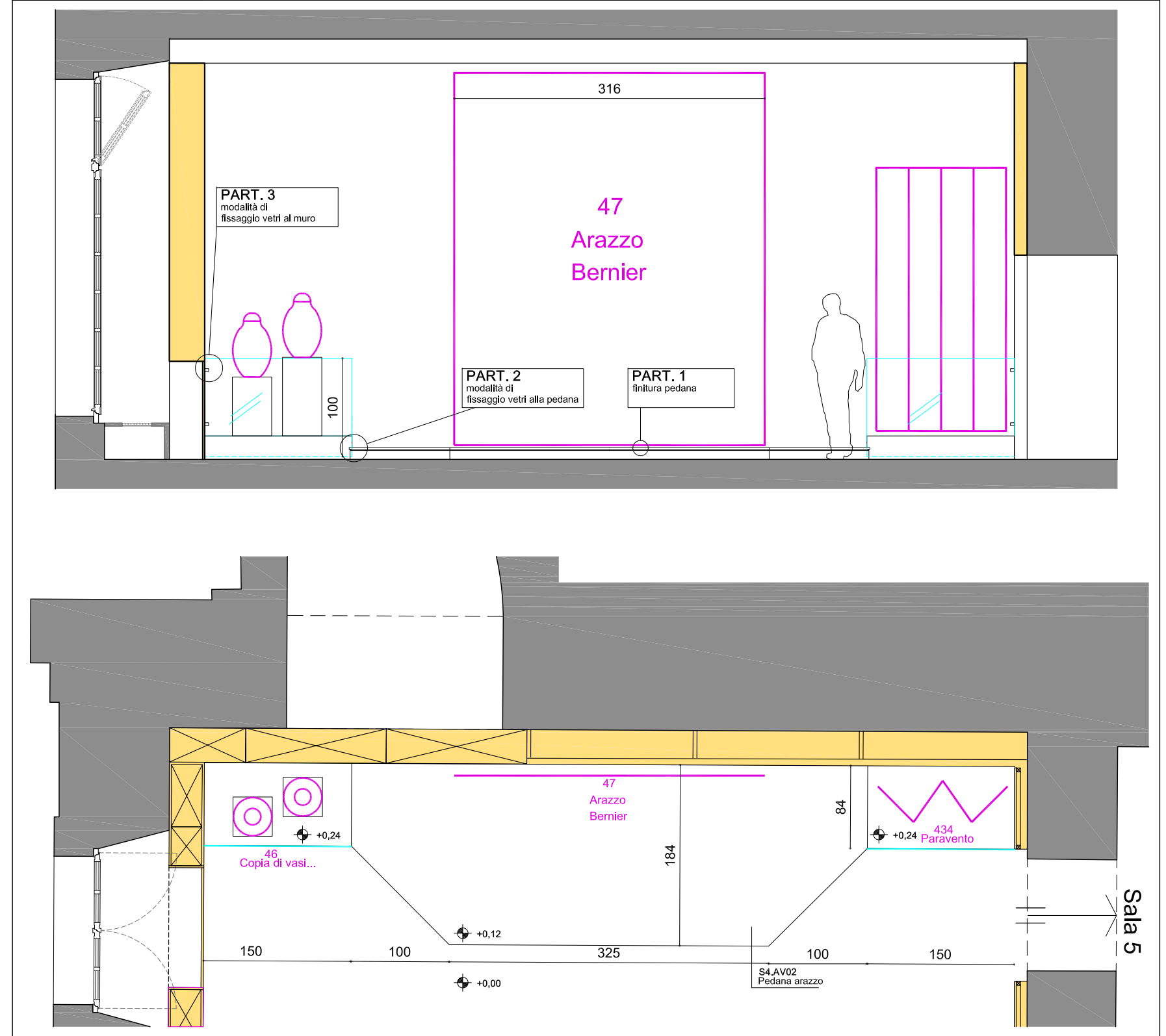
S4.AV02 Pedana arazzo con vetri di protezione laterali
