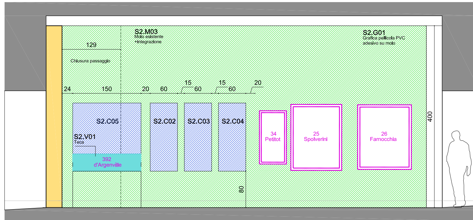
Parete 3
