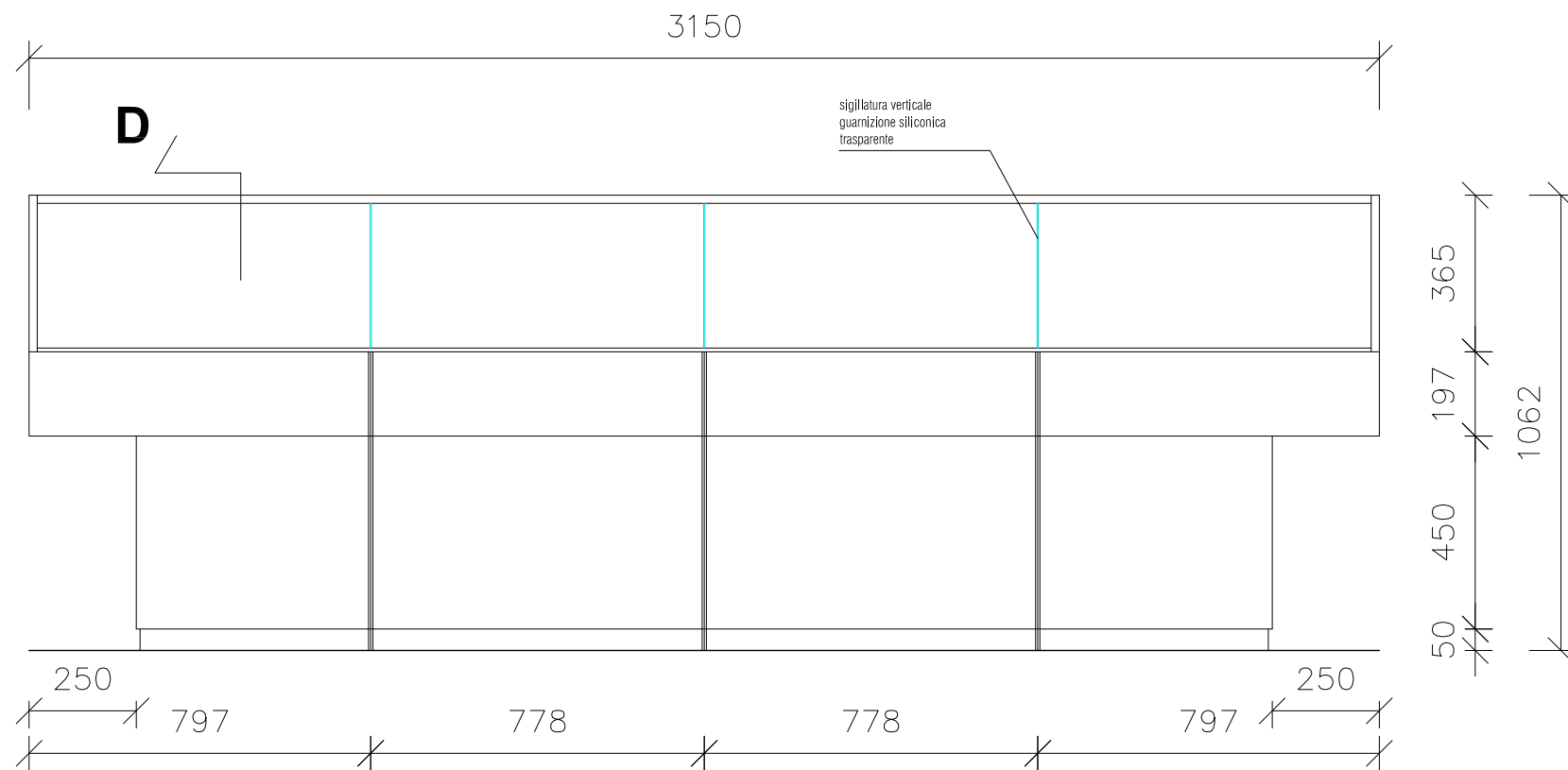
PROSPETTO FRONTALE
