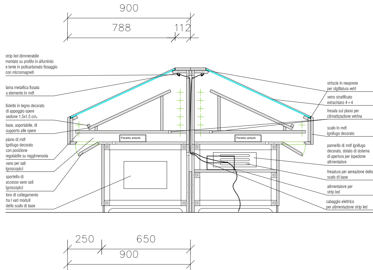
SEZIONE A
