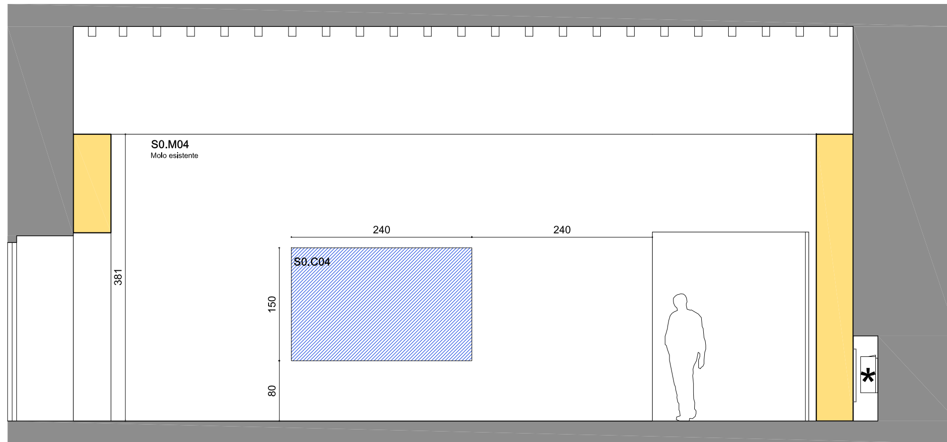
Parete 4
