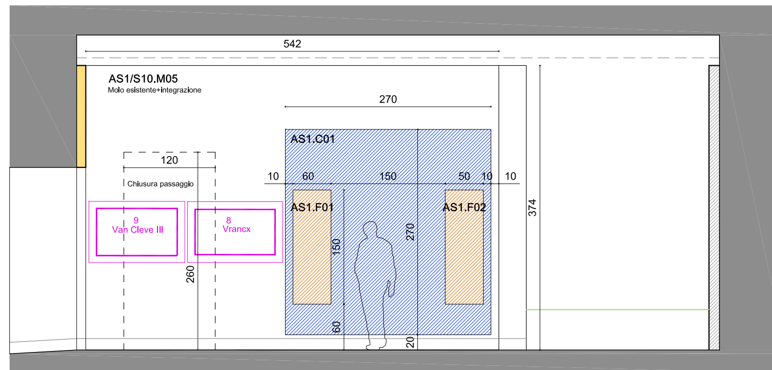
Parete 4
