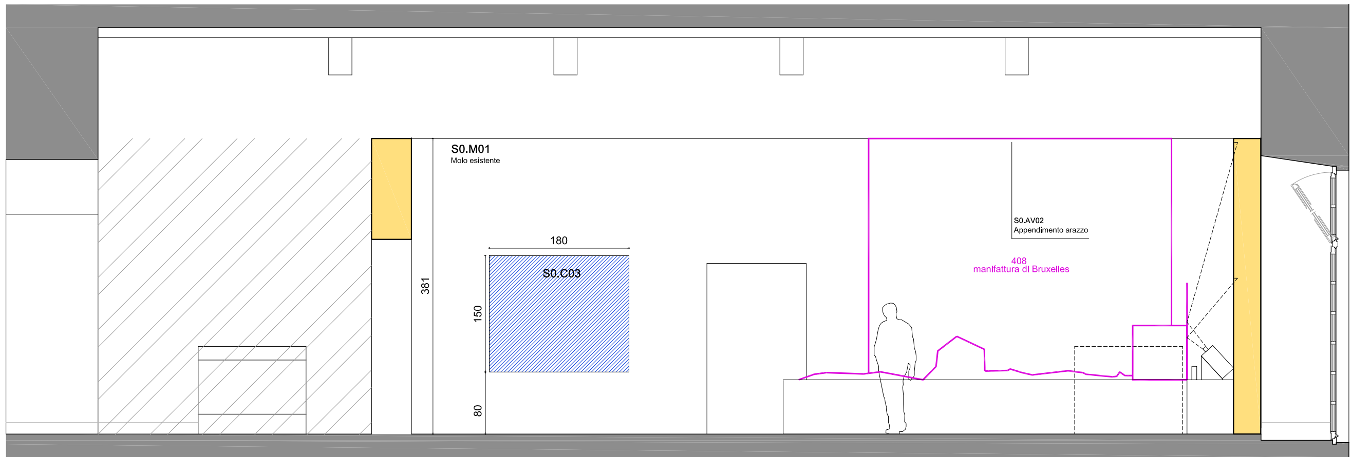
Parete 1
