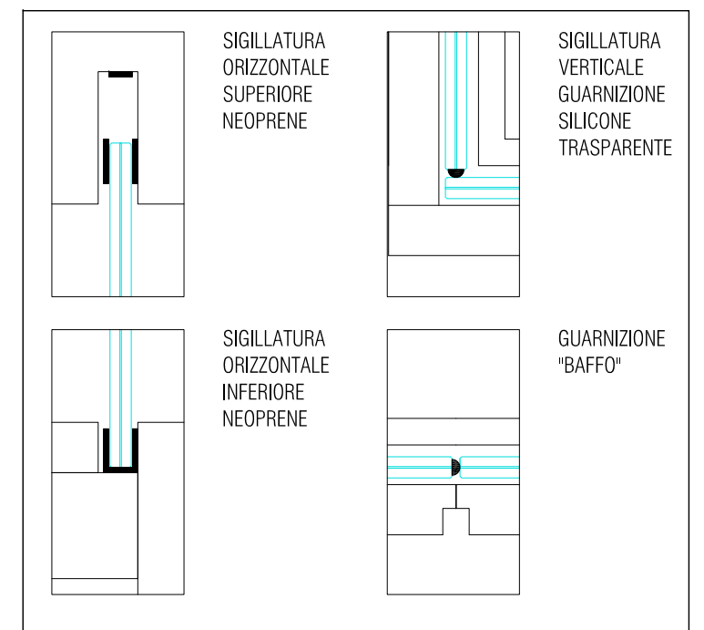
DETTAGLIO SIGILLATURA VETRI
