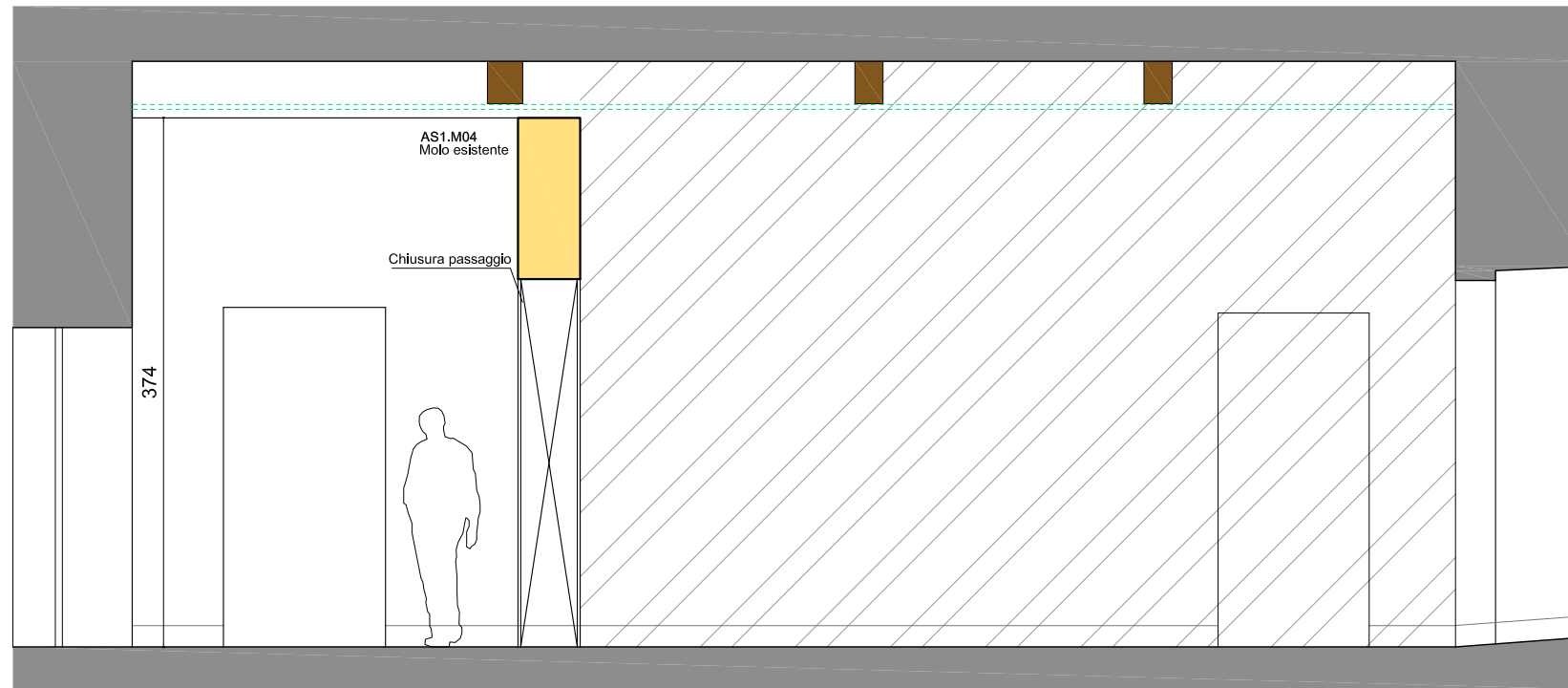
Parete 3
