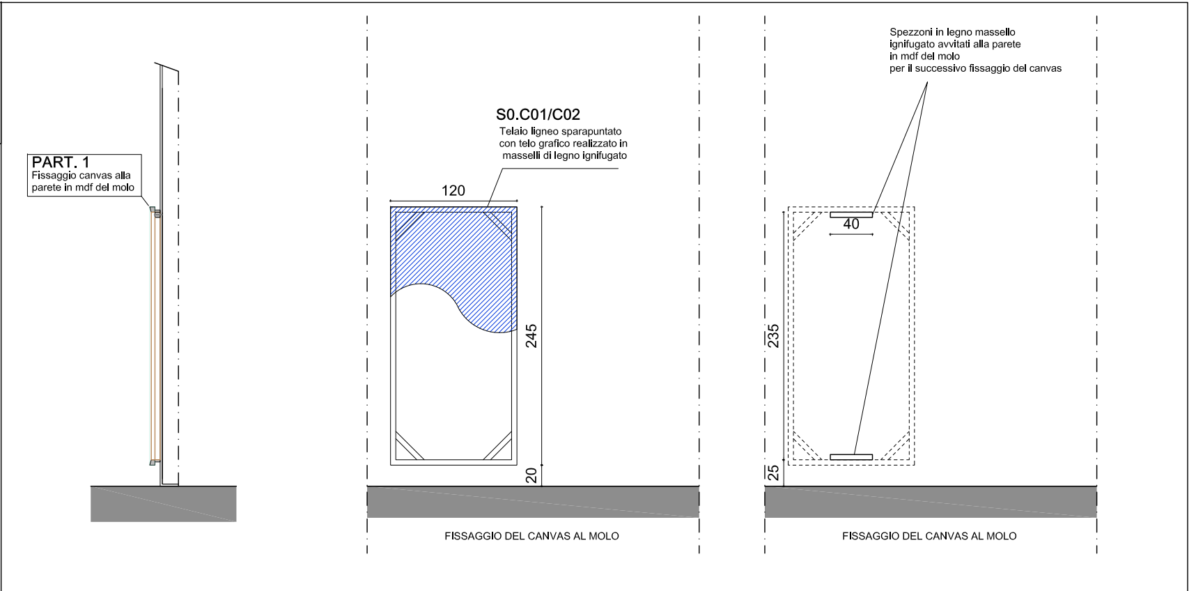
S0.C01/C02 Telaio ligneo sparapuntato con telo grafico realizzato in masselli di legno ignifugato
