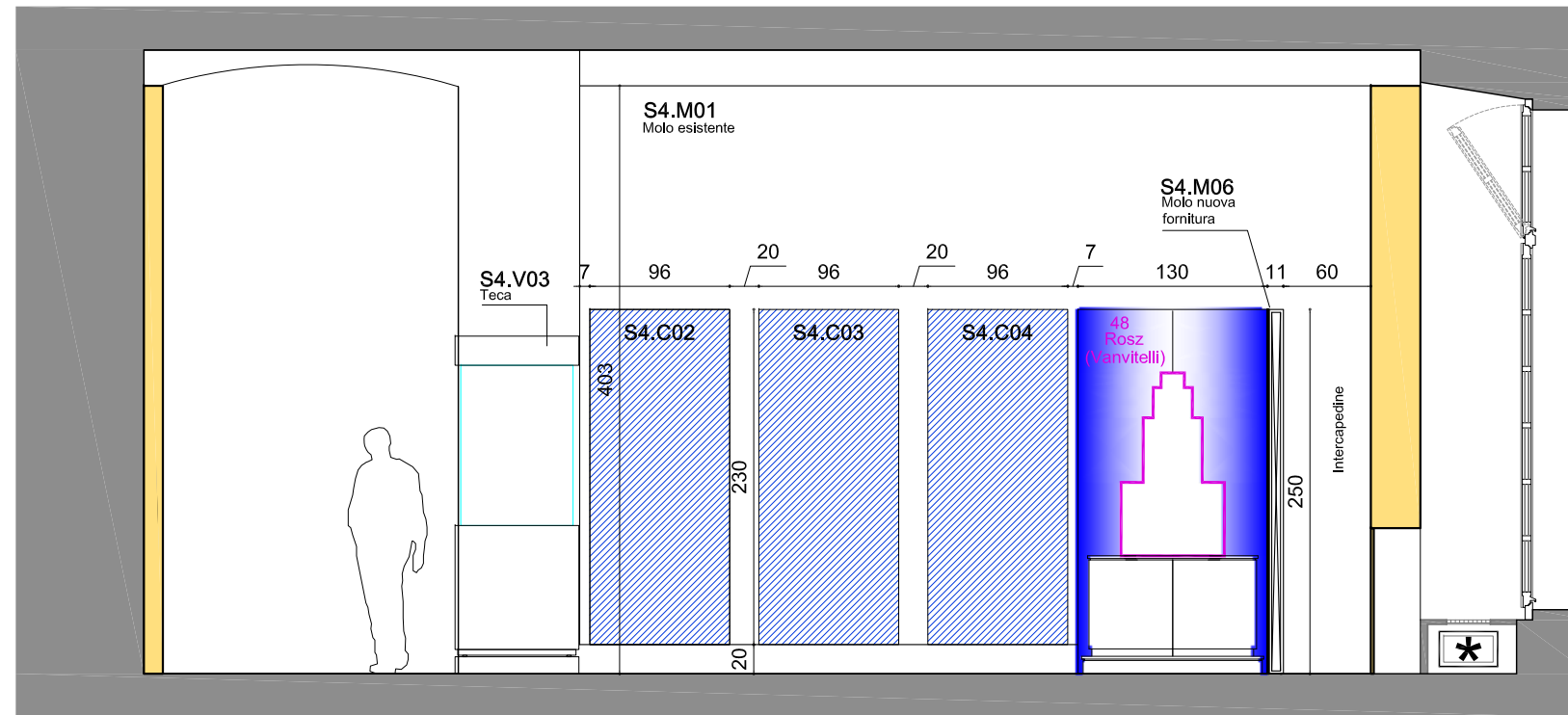
Parete 1
