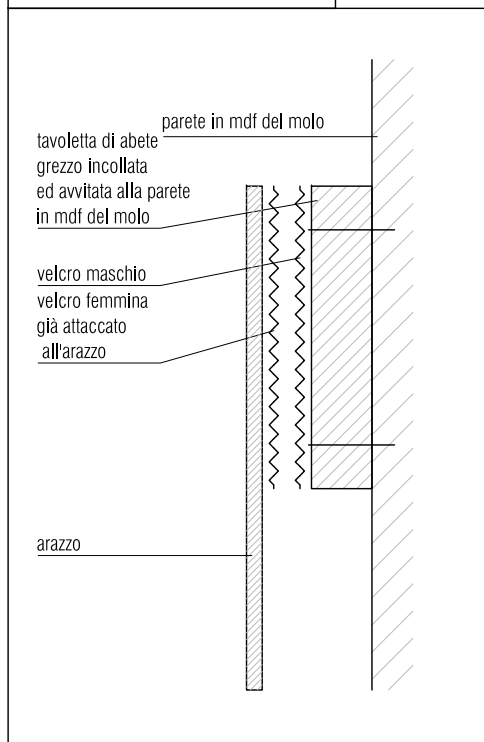
S4.AV06 Appendimento arazzo
