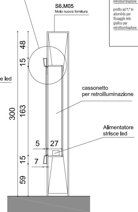
SEZIONE
