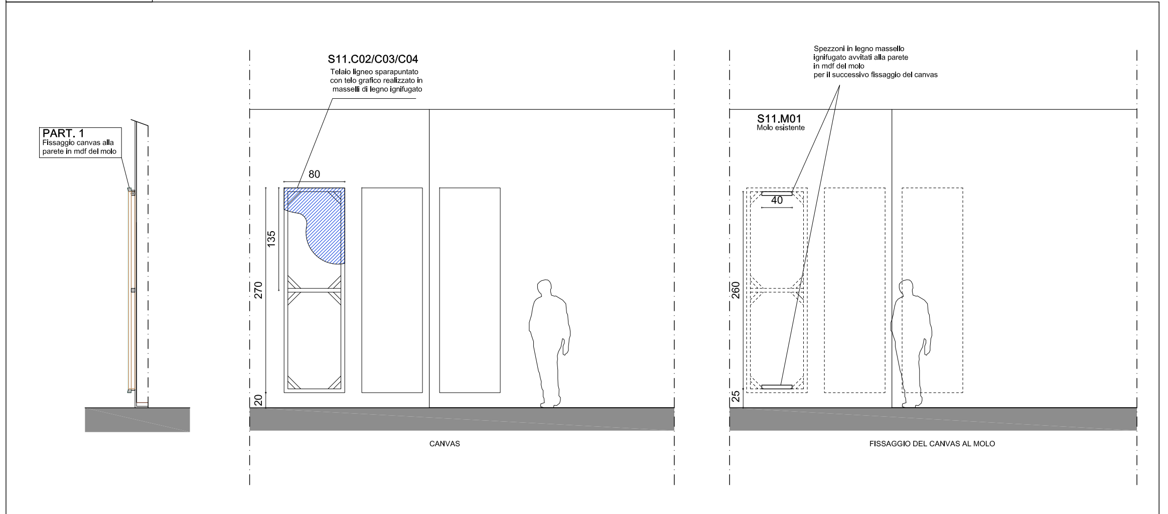
S11.C02/C03/C04 Telaio ligneo sparapuntato con telo grafico realizzato in masselli di legno ignifugato
