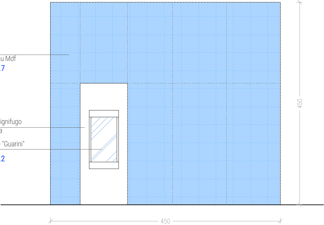
PROSPETTO - scala 1:50
