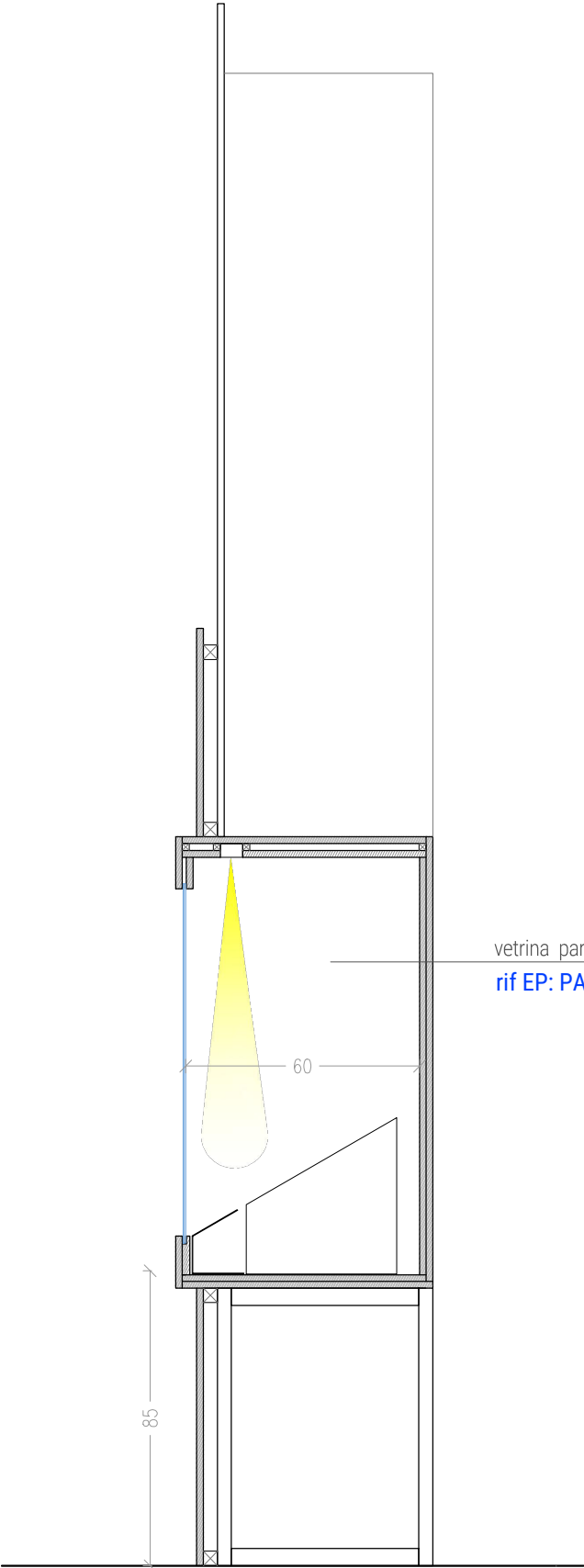
SEZIONE - scala 1:20
