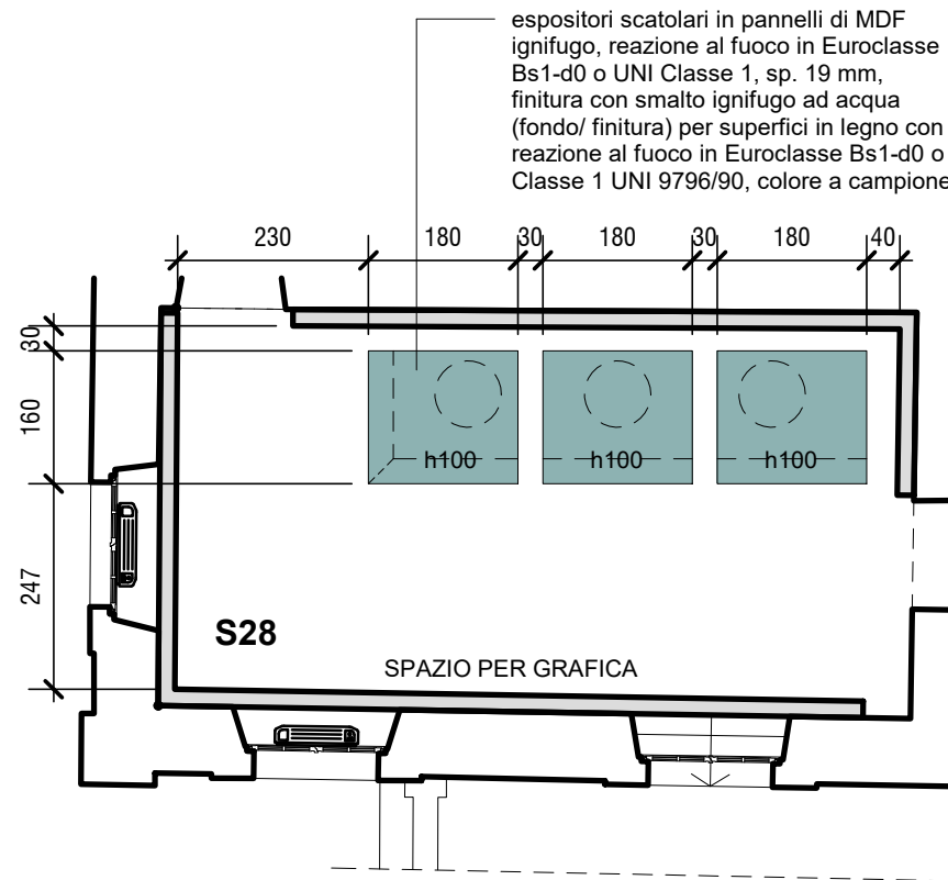
Pianta Sala S28 1 : 100
