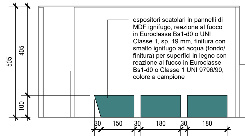
Sala S28 - Sezione longitudinale 1 : 100
