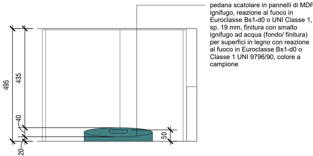
Sala S30 - Prospetto pedana 1 : 100
