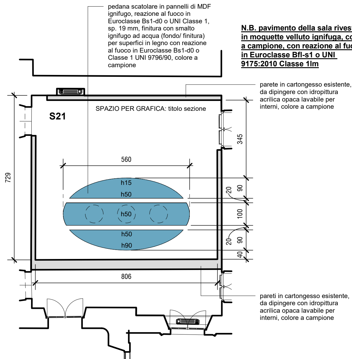
Pianta Sala S21 1 : 100
