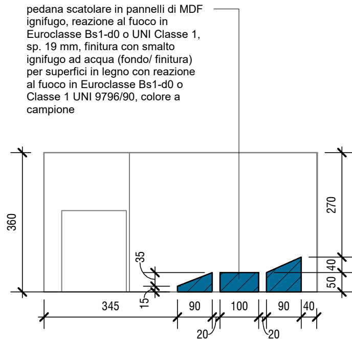
Sala S21 - Sezione trasversale 1 : 100
