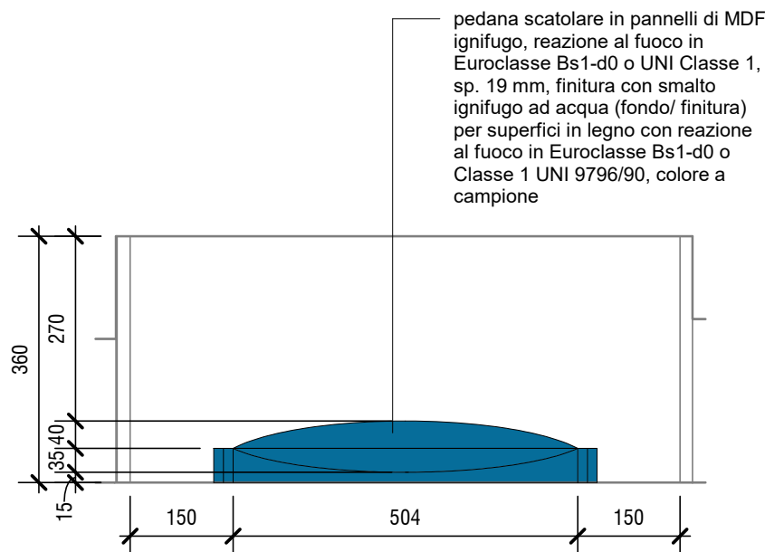
Sala S21 - Sezione longitudinale 1 : 100
