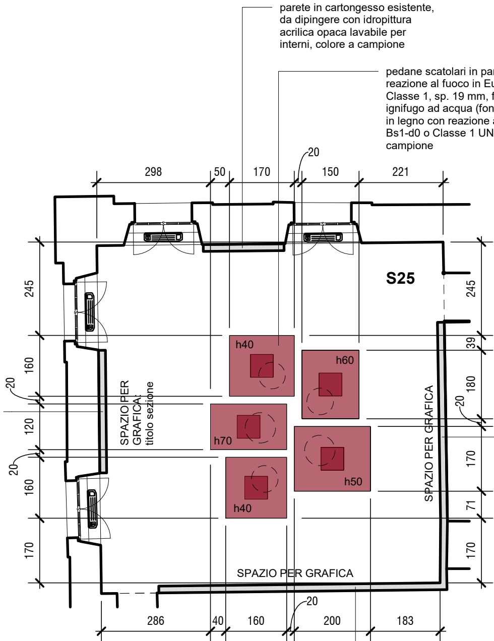
Pianta Sala S25 1 : 100
