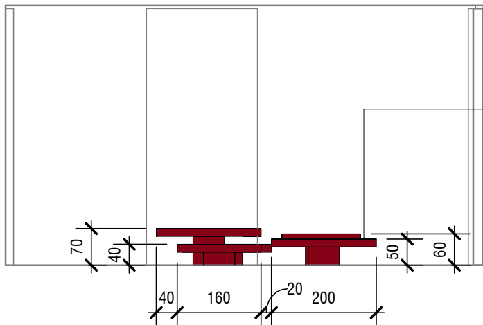
Sala S25 - Sezione trasversale 1 : 100
