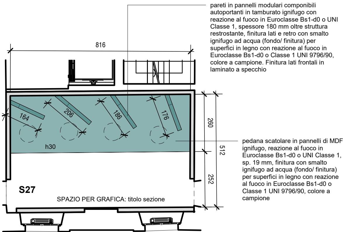
Pianta Sala S27 1 : 100
